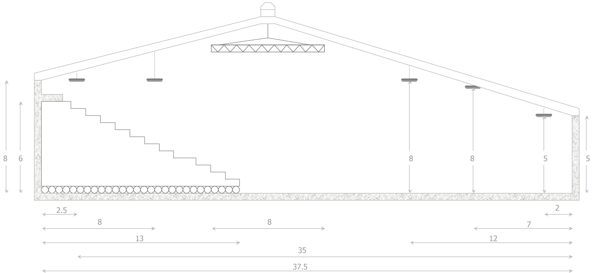
SEZIONE - VISTA LATO HOTEL - TRIBUNE APERTE
